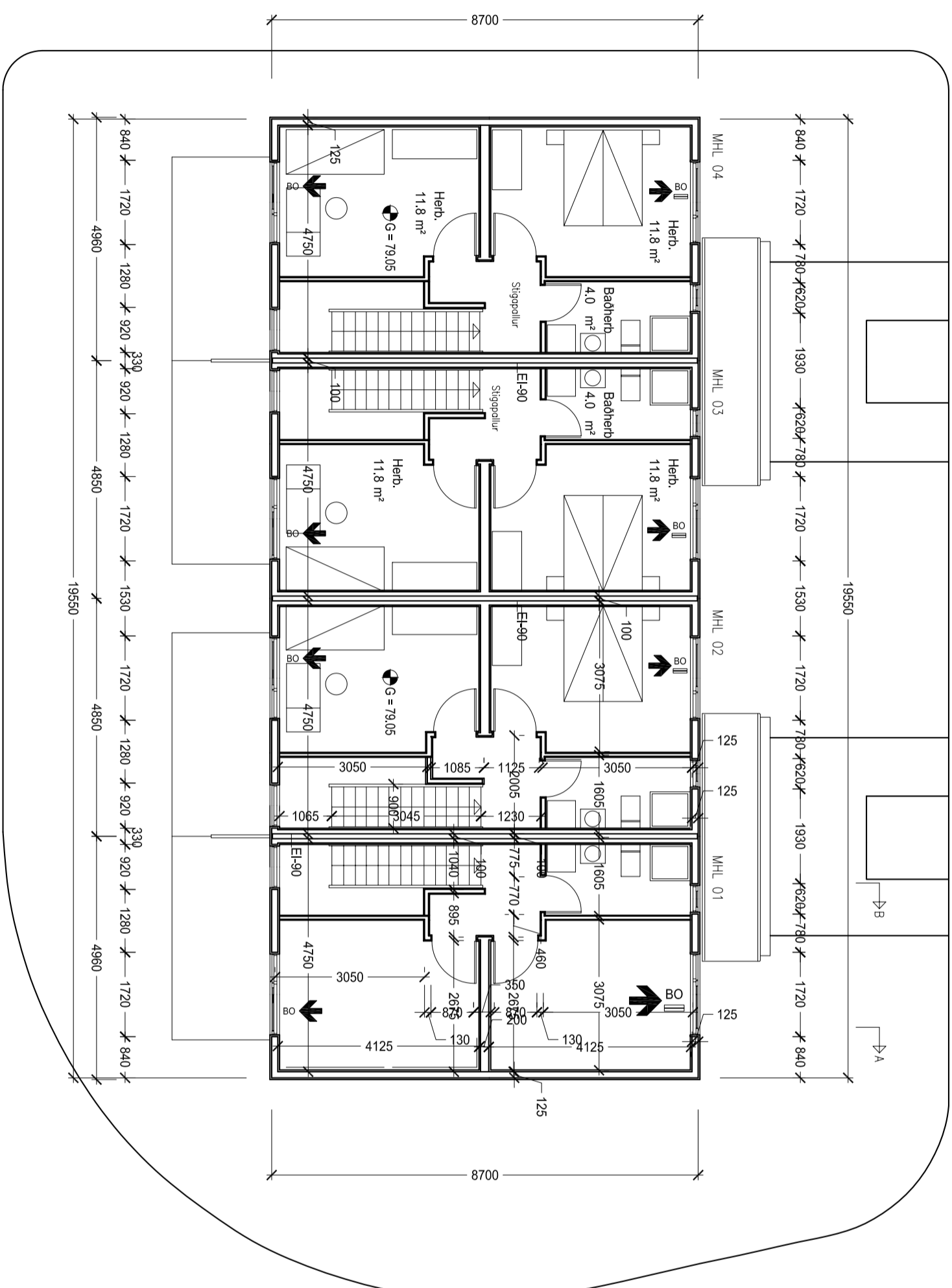
Grunnmynd Eflihæðar 1:100
