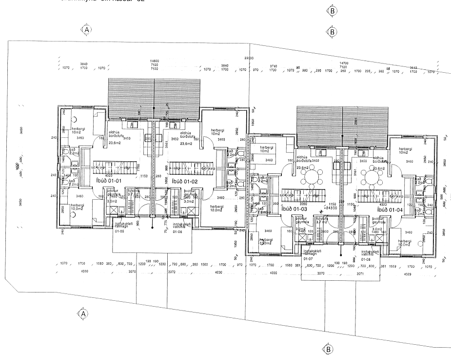
Grunnmynd jarðhæðar 01
